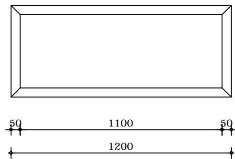
Bovenaanzicht
