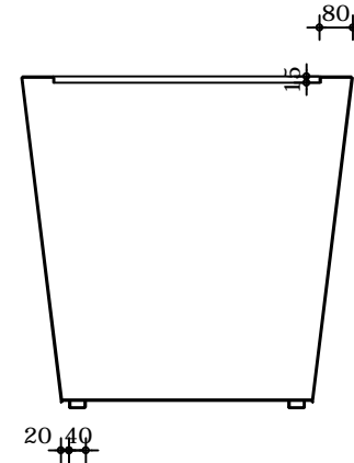
Verticale doorsnede
