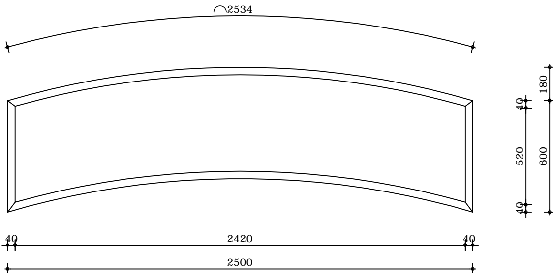
Bovenaanzicht
