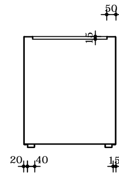
Verticale doorsnede
