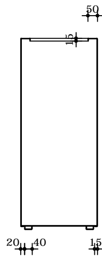
Verticale doorsnede
